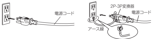
(a) 接地極付きコンセント(3穴)への接続 (b) アース端子付きコンセントへの接続
